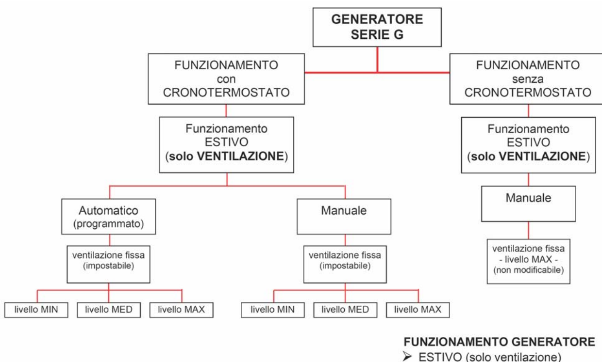
Figura 13 – Funzionamento estivo.
