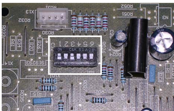
Figura 40 – Posizione minidip scheda.
