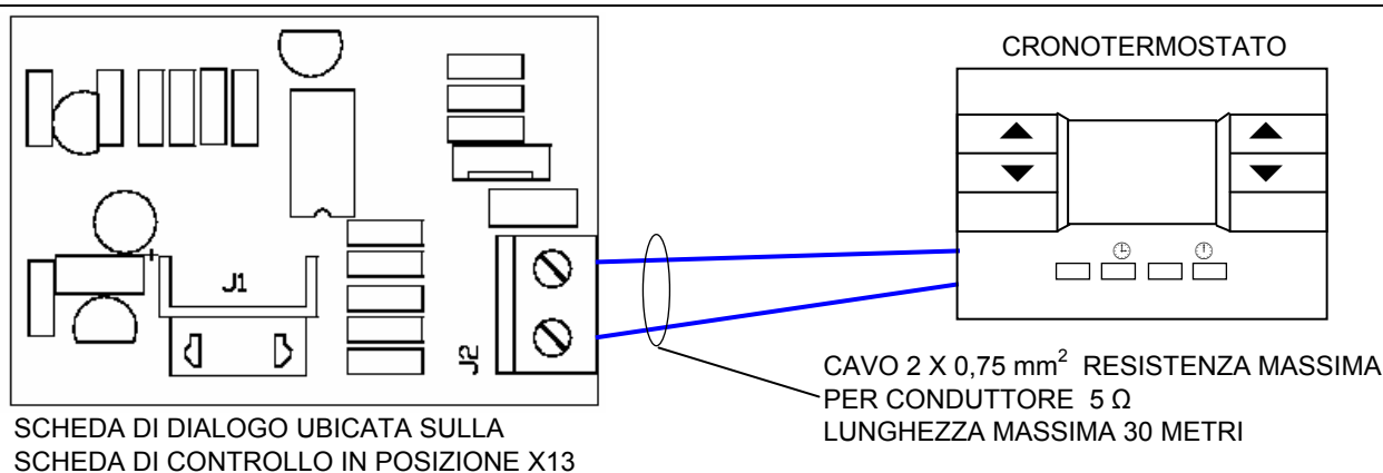
Figura 32 – Collegamento cronotermostato e scheda di dialogo.
