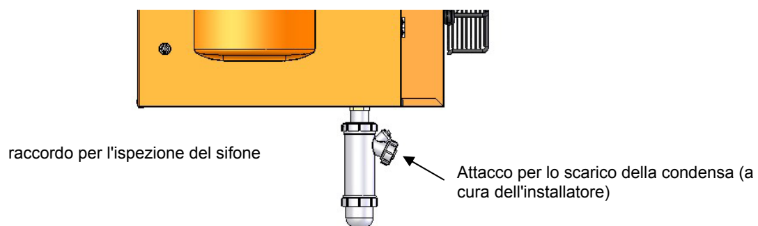
Figura 31 – Particolare dell'installazione sifone scarico condensa.
