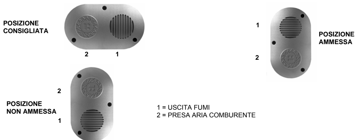
Figura 17 – Posizione terminale a parete.
