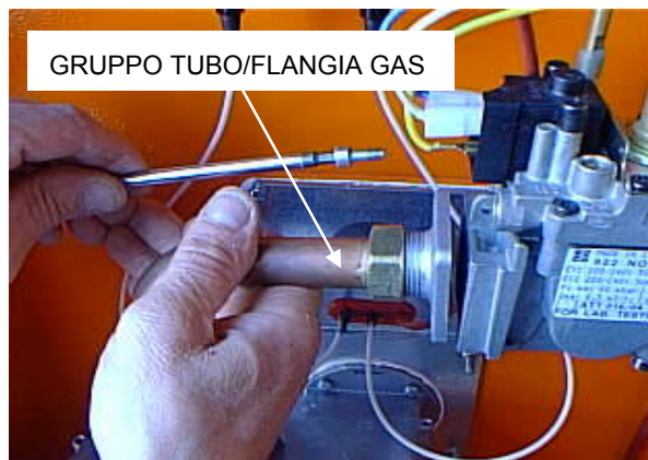
Figura 37 – Gruppo tubo/flangia gas.
