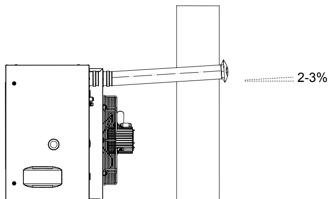
Figura 16 – Contropendenza tubi orizzontali.
